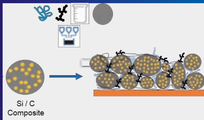
Formulation d'une anode à base de silicium - Crédits : Nanomakers
