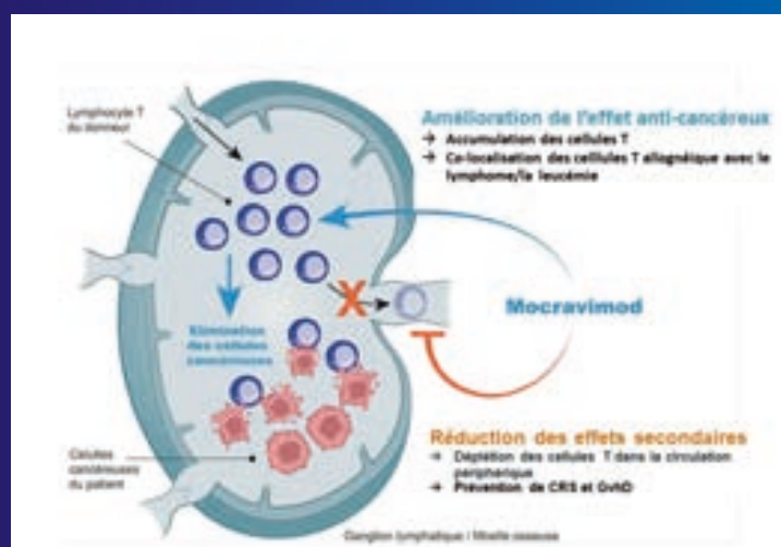
Mécanisme d'action de mocravimod - © Priothera SAS
