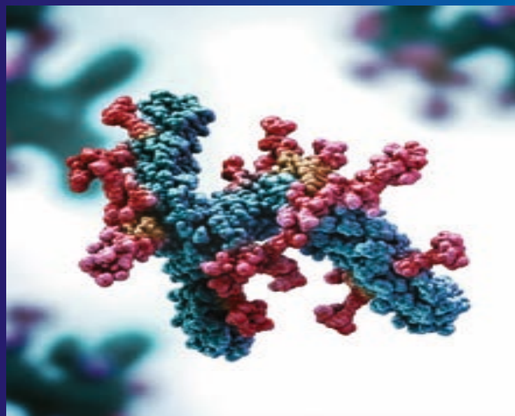
Représentation d'un anticorps couplé à une drogue Source StarkAge Therapeutics
