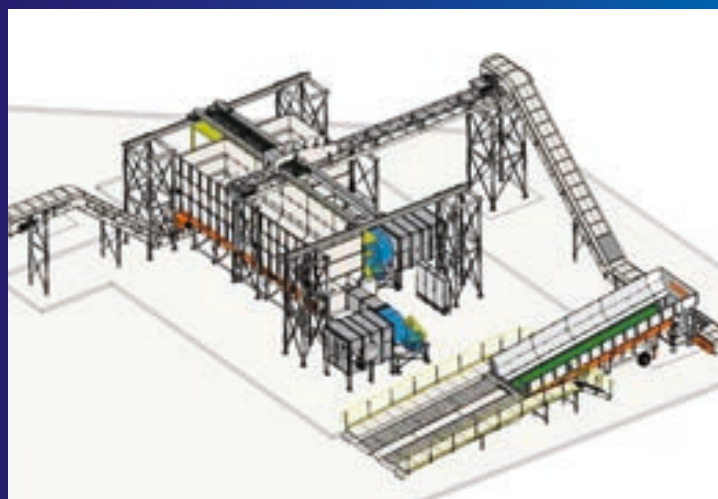
Vue d'ensemble de la conception du prototype Crédit : Ets Jules N'Haux & Fils
